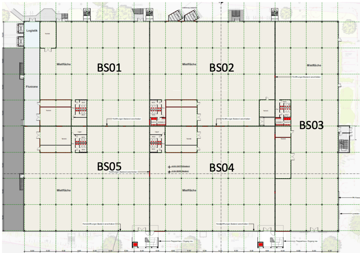
Grundriss EG
