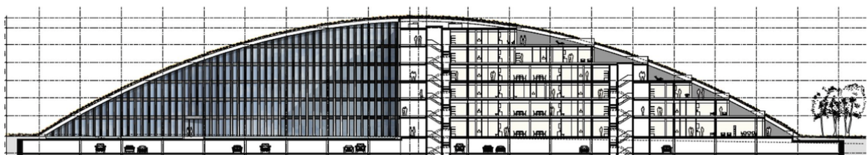
Seitenschnitt Gebäude
