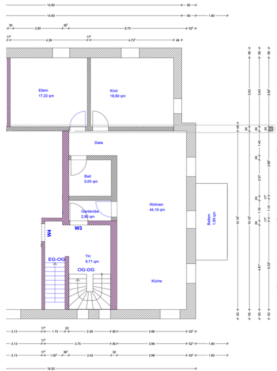
Grundriss Wohnung
