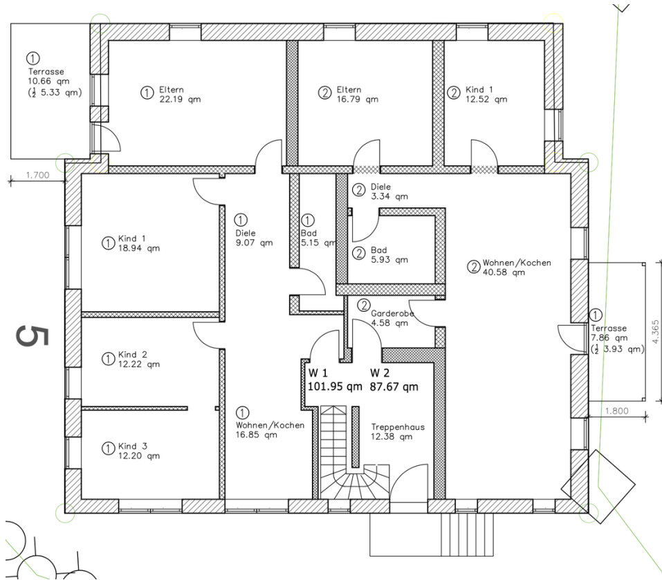
Grundrissplan - Wohnung 2
