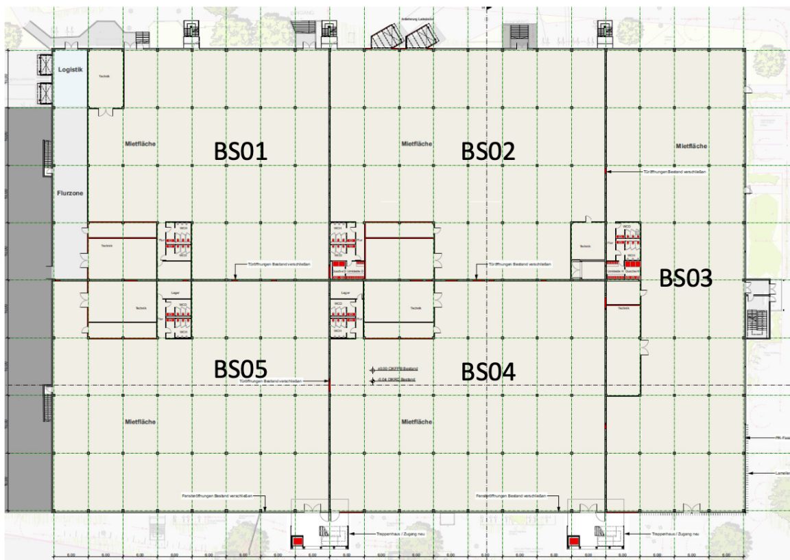
Grundriss EG
